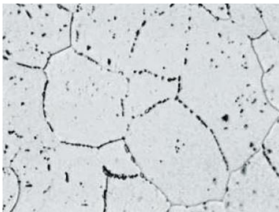
ABBILDUNG 63 | Interkristalline Korrosion
