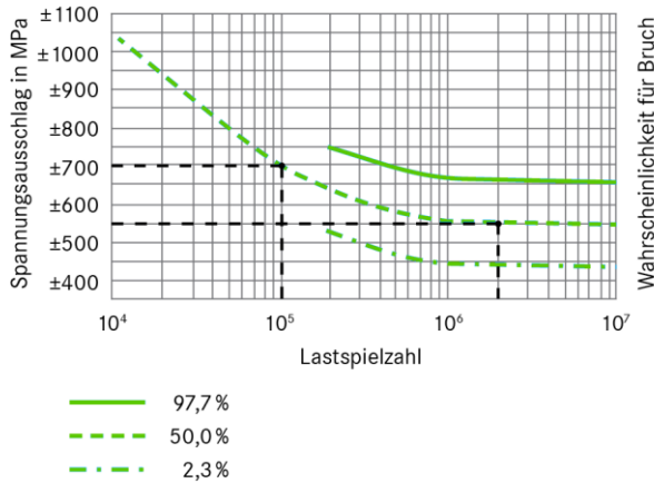
ABBILDUNG 37 | Biegewechselspannung
