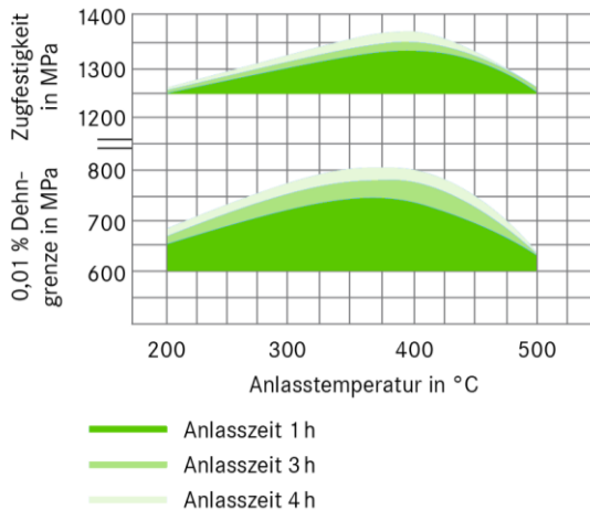
ABBILDUNG 49 | Einfluss Anlasstemperatur
