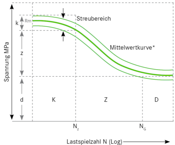
ABBILDUNG 31 | Wöhlerschaubild / Prinzip
