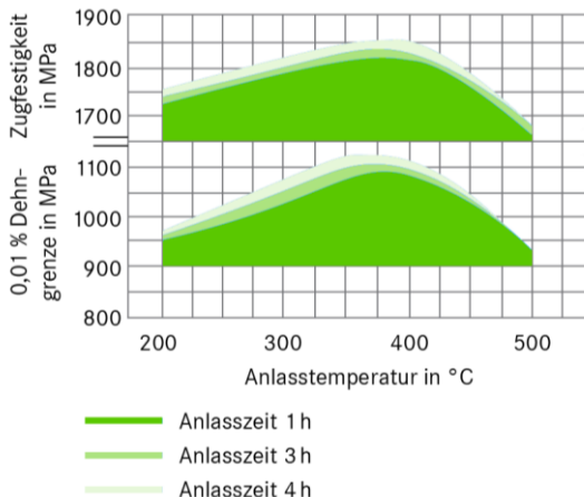
ABBILDUNG 50 | Einfluss Anlasstemperatur
