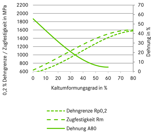
ABBILDUNG 22 | Mechanische Werte 1.4310FM
