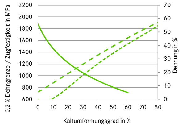
ABBILDUNG 23 | Mechanische Werte 1.4310FC
