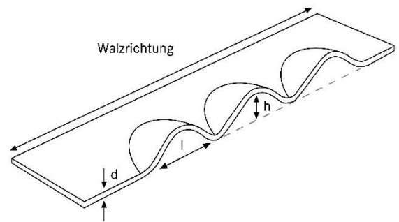
ABBILDUNG 2 | Kantenwelligkeit
