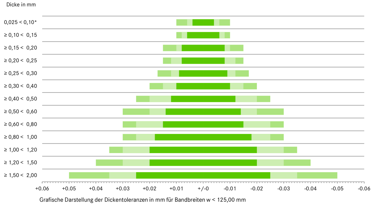
Abbildung 1 | Banddickentoleranzen in mm
