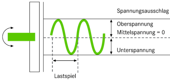
ABBILDUNG 36 | Biegewechselspannung
